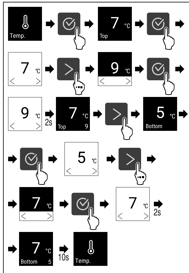
Fig. 31 Промяна на температурата от 7 °C на 9 °C и от 5 °C на 7 °C*
